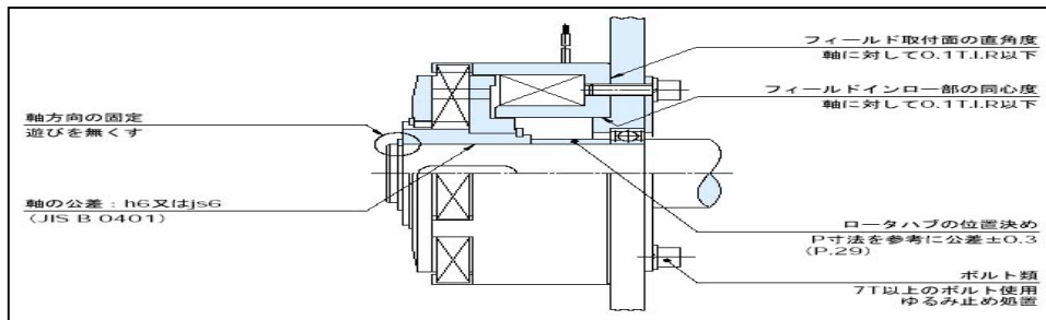
그림3 MDB형 브레이크 기본취부 예
