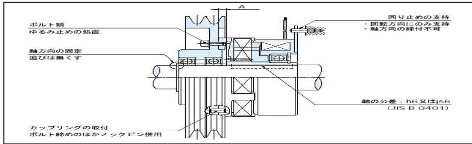
그림 2 MDC형 클러치의 기본 취부예
